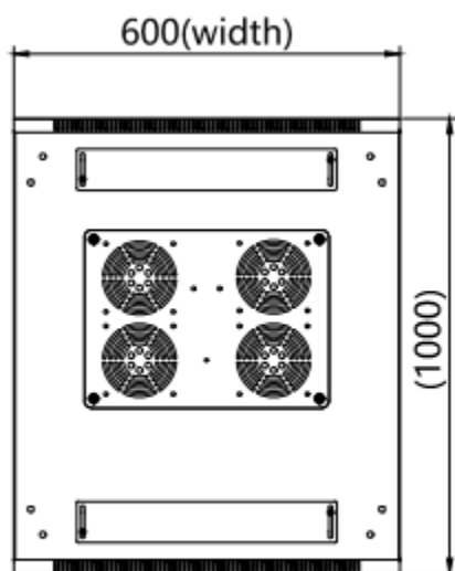
TOP
